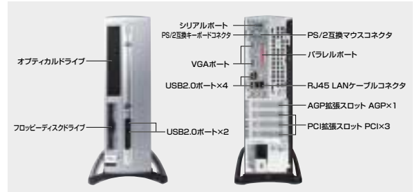
前・背面図
