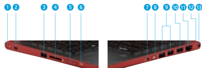
左側面
