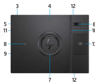
タブレット背面 HP Engage Go 13.5" Convertible System with Grip
